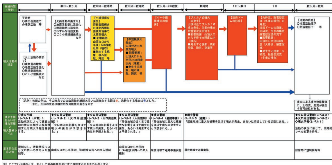
図 5 那須岳火山の噴火シナリオとその防災対応 噴火活動の推移での必要とされる防砂対応などを噴火シナリオにより策定した。 Fig. 5 Eruption scenario and Disaster prevention measures of Nasu volcano. Disaster prevention measures were referred from eruption scenario.
