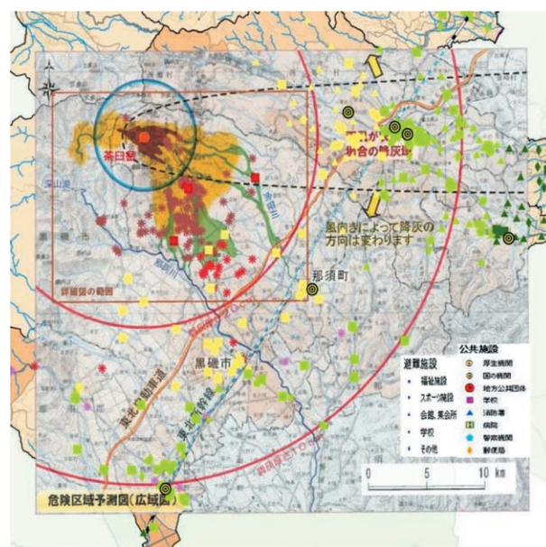
図8 那須岳周辺地域の噴出物想定分布域と公共施設・宿泊施設の分布
