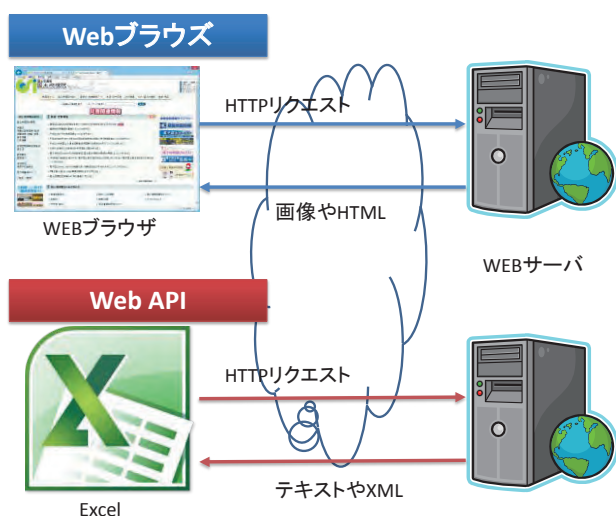
図-2 Web ブラウズと Web API
