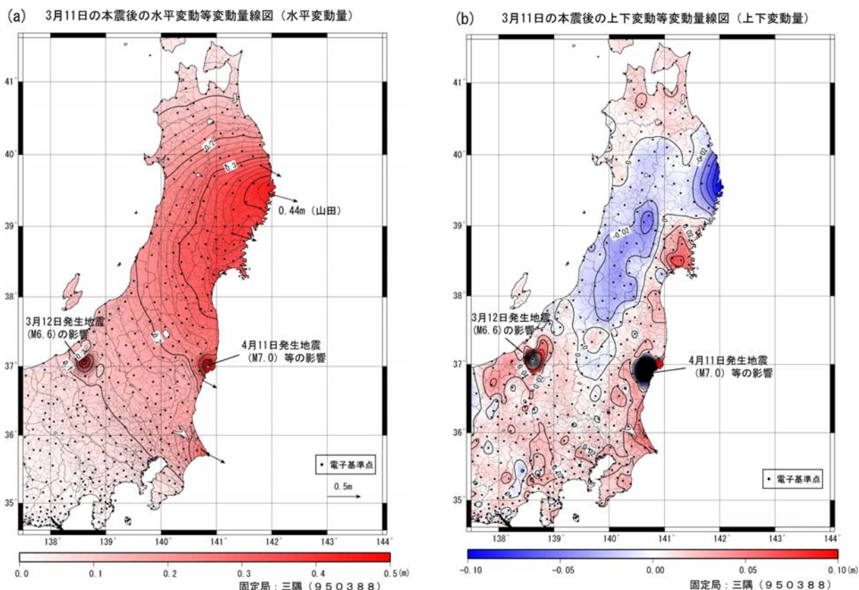
図－2 地震後の地殻変動等変動量線図（3月11日－4月17日：Q3解及びR3解）(a) 水平変動量 (b) 上下変動量
