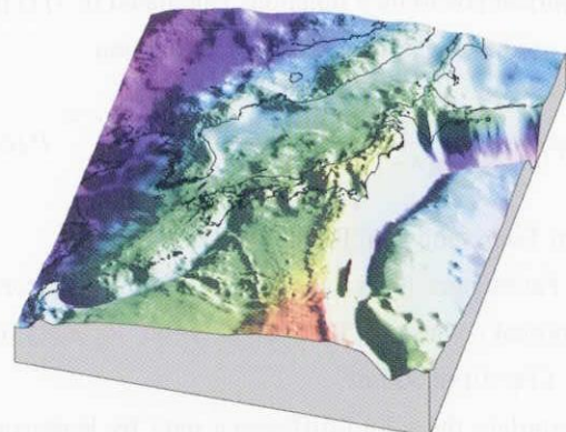
Fig. 5 Relief map of JGEOID2000.
