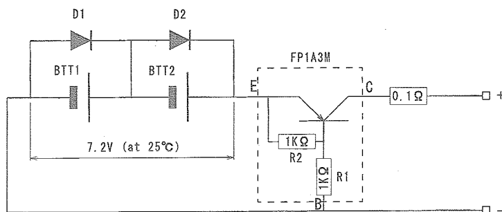
図 1 トランジスタ FP1A3M を通って電流が漏洩した。60 日間の輸送中、3.6mA が常時流れることになってしまった。
