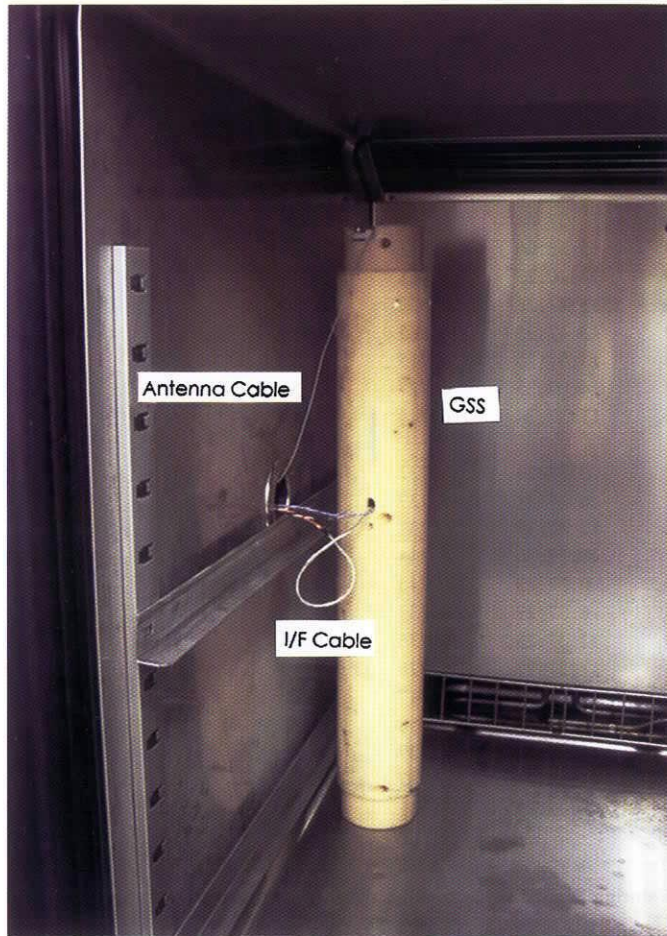
図 5 実験風景。(a) 測定に関係した機器類。(b) GSS はタバイ PL-3FPW の恒温槽に実際の設置姿勢で入れ、 -15^{\circ}\text{C} に設定した。無線アンテナは筐体上部から、ケーブルで延長し、側面の孔から外へ引き出した。GSS の中間から出ているケーブル 2 本は I/F 回路につながっている。
