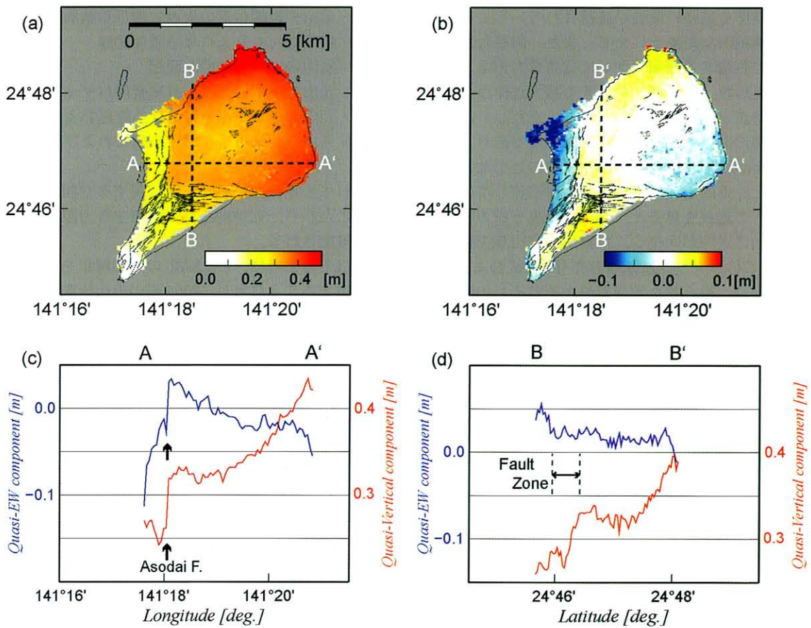
図 7 干渉ペア A3, D1, D2 から求めた 2 次元地殻変動。(a)大八木・井口(1985)による断層分布と重ねて示した準上下成分。(b)大八木・井口(1985)による断層分布と重ねて示した準東西成分。(c)図 7(a)および(b)の A-A'における準上下成分(赤線)と準東西成分(青線)のプロファイル。(d)図 7(a)および(b)の B-B'における準上下成分(赤線)と準東西成分(青線)のプロファイル
