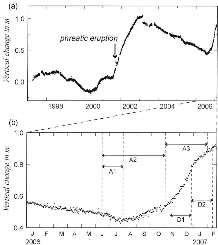
図 2 (a) 電子基準点「硫黄島 1」の上下変位を示す時系列。基準点は電子基準点「母島」である。(b)2006 年以降の拡大図。矢印は、本研究で解析した干渉ペアの期間を示す。矢印と共に示す番号は、表 1 に示す干渉ペア番号に対応する。
