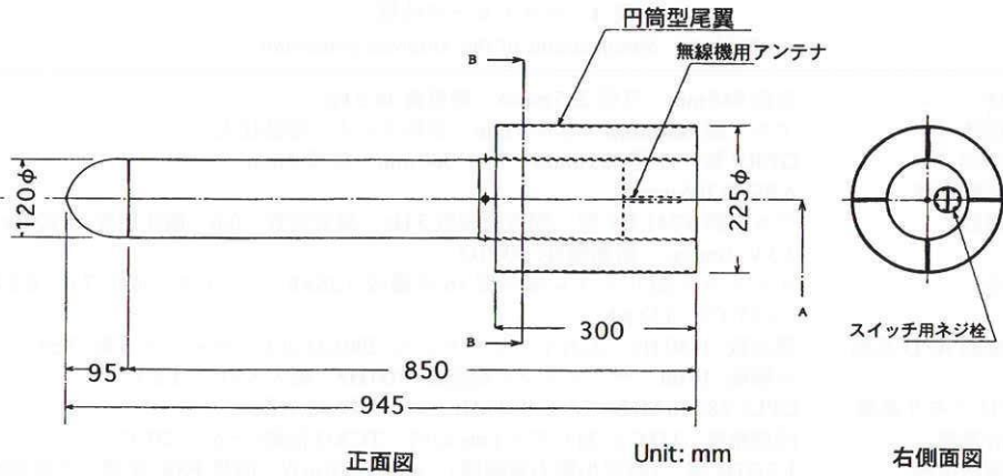
図1 ペネトレータ平面図
