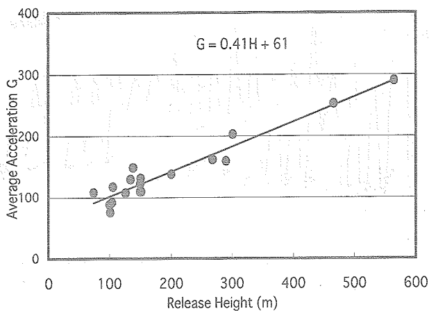
図10 投下高度に対する着地時の平均衝撃加速度
