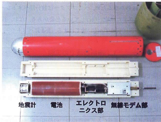
図2 開発された南極ペネトレータの内部
