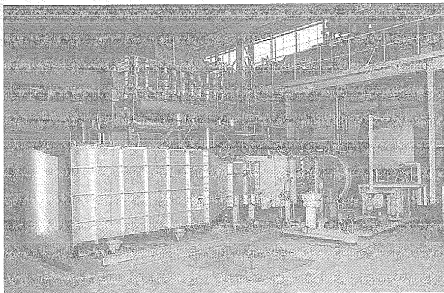
図4 伝熱特性検証設備
