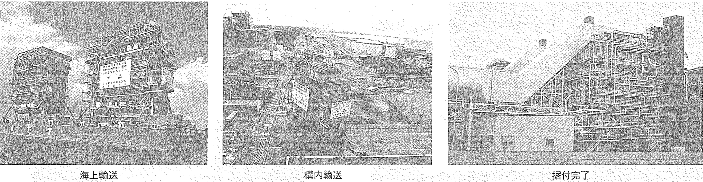
図6 大型モジュールによる輸送・据付
