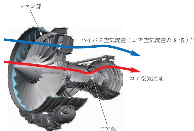
第 3 図 バイパス空気とコア空気の流れ Fig. 3 Bypass and core flow
