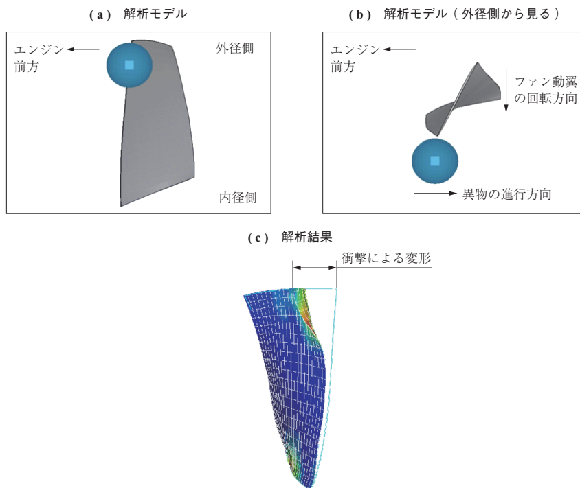
第 5 図 異物吸込みに対するファン動翼変形の変位解析例 (10) Fig. 5 Transient analysis of deformation of fan blade impacted by foreign object (10)
