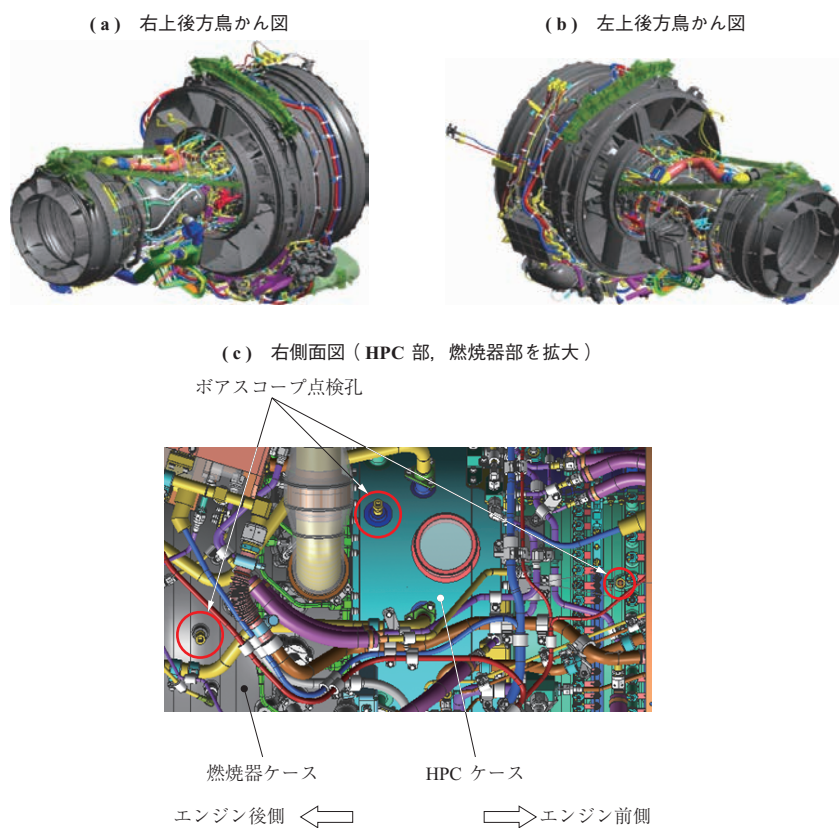
第 15 図 三次元 CAD を使用した艤装設計 Fig. 15 External design with 3D-CAD
