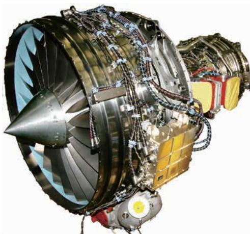
第 1 図 F7-10 エンジン外観 Fig. 1 External view of the F7-10 engine
