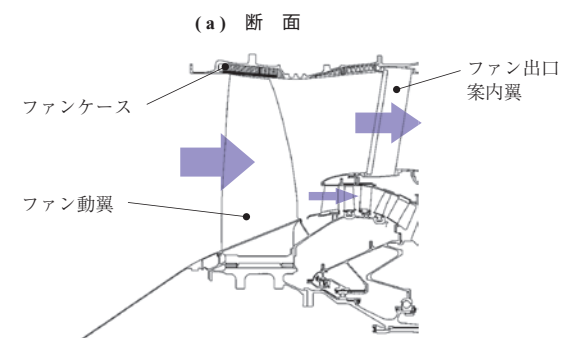
第 6 図 ファン部 Fig. 6 Fan section
