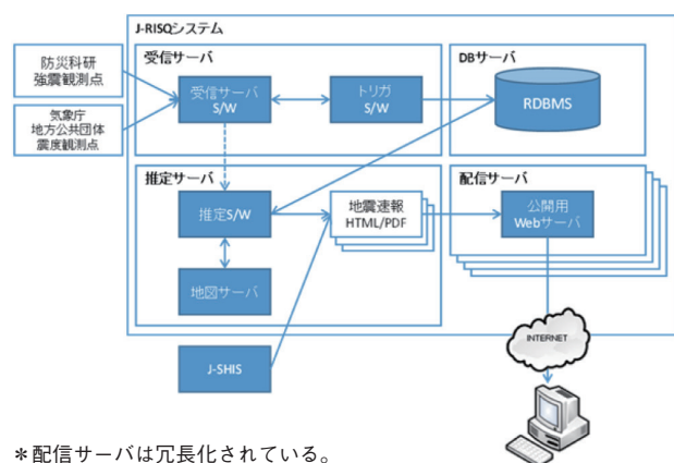
図1 J-RISQのシステム構成図
