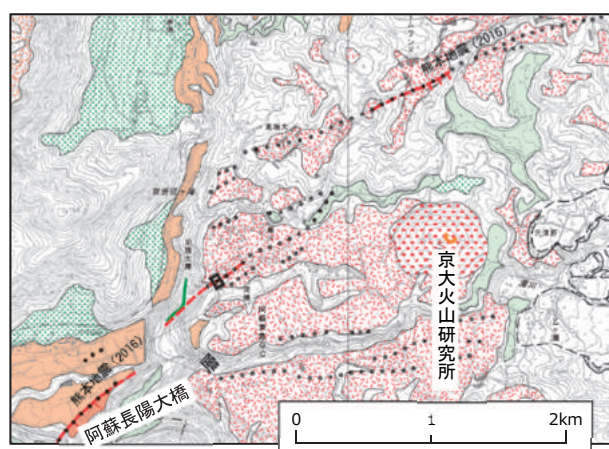
図-6 阿蘇カルデラ内に現れた地震断層と新たに確認された活断層（1:25,000 活断層図「阿蘇」の一部・南阿蘇村河陽周辺）
