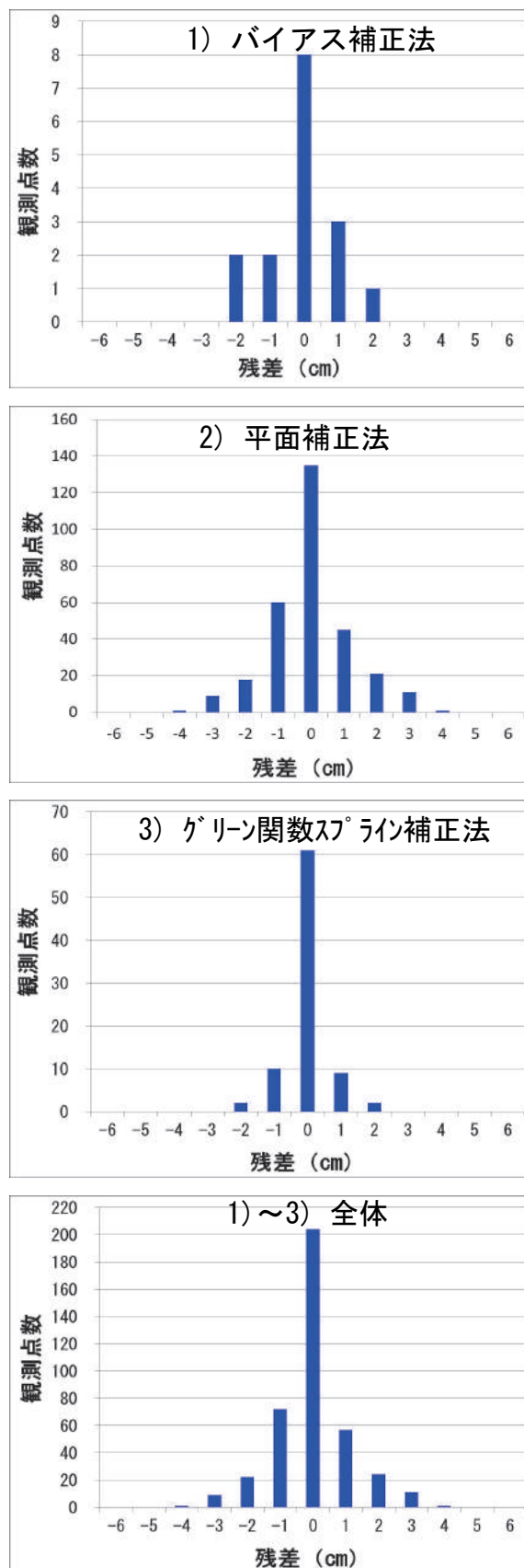
図-6 各補正法におけるジオイド高データとジオイ・モデルとの差の度数分布
