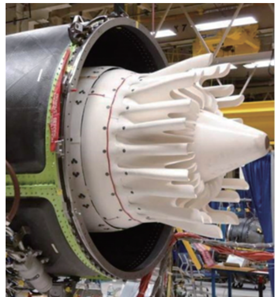
第 11 図 CMC ミキサノズル Fig. 11 CMC mixer nozzle
