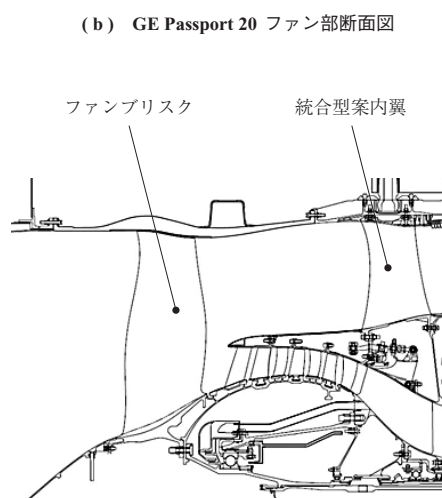
第 7 図 ファンブリスクと統合型案内翼 Fig. 7 Fan blisk and integrated guide vane
